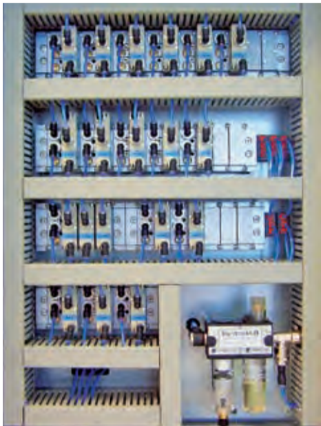
Individueller Service: Fey Schaltschrank nach Kundenspezifikation.
